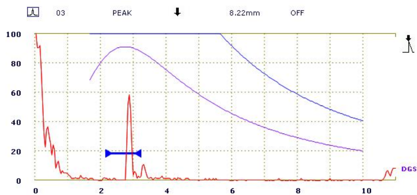
Obr. 1 Hore – indikácia neprievaru, dolu - indikácia pretečeného zvaru (kvapľa) v koreni V zvaru potrubia \varnothing 158 \times 9 mm pri skúšaní uhlovou sondou 70^\circ . (Rozsah časovej základne 100 mm).
