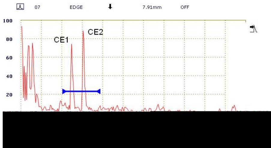
Obr. 3 Kolatelárne echá CE1 a CE2 od koreňového neprievaru vo V zvare potrubia \varnothing 158 \times 9 mm.
